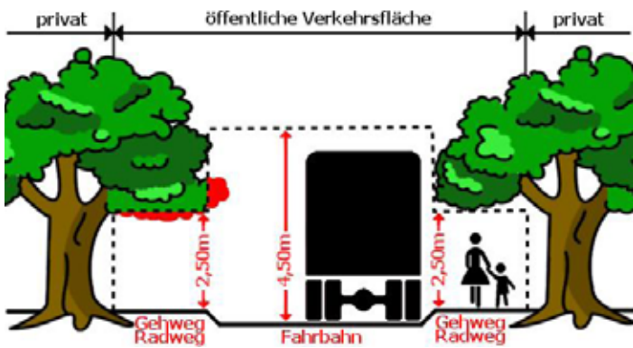
Grafische Darstellung des Lichtraumprofils für Radwege und Fahrbahn
